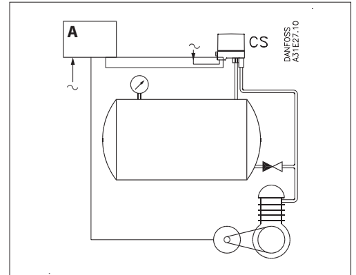
Exemple 2 Régulation d'un compresseur à air au moyen d'un interrupteur de pression type CS avec soupape de décharge. Remarquez le clapet antiretour entre la conduite d'égalisation et le réservoir.
