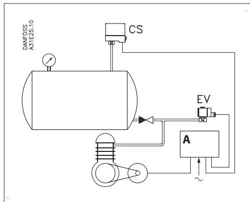
Exemple 3 Régulation d'un compresseur à air au moyen d'un interrupteur de pression type CS. Pour les installations exigeant une égalisation rapide de la pression, il est recommandé de monter une électrovanne EV210B 3B.
