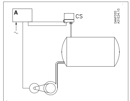
Exemple 4 Régulation d'une pompe centrifuge au moyen d'un interrupteur de pression type CS par l'intermédiaire d'un coupleur étoile-triangle automatique, d'un discontacteur ou similaire.
