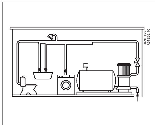
Exemple 5 Pressurisation des installations dans les immeubles. La commande arrêt/marche de la pompe est assurée par un interrupteur de pression CS
