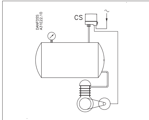
Exemple 1 Régulation d'un compresseur à air au moyen d'un interrupteur de pression type CS.
