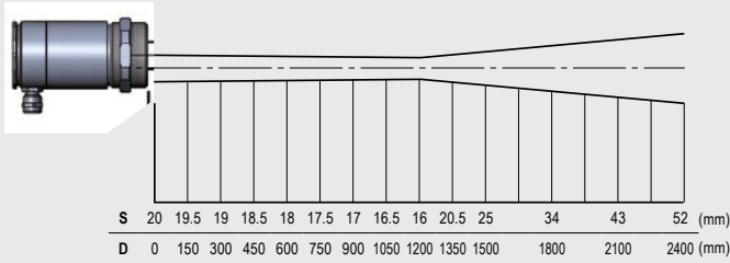
SF optics 75:1
