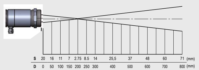
CF3 optics 75:1
