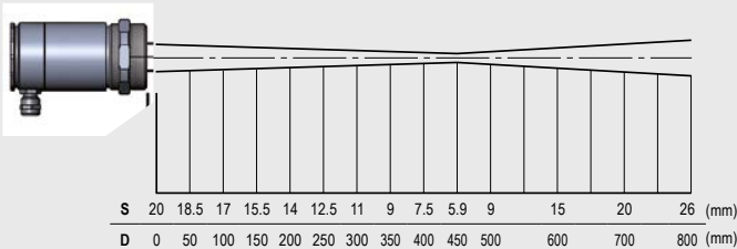
CF4 optics 75:1
